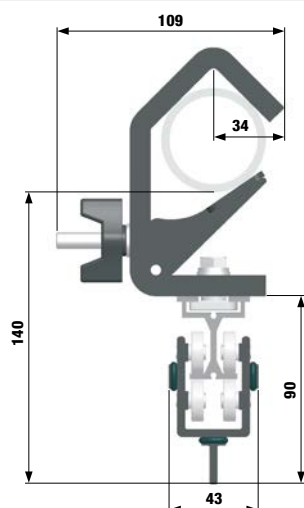
Vorderansicht / Vue en coupe / End View
