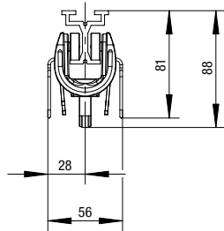
2-Rad-Laufwagen + Vorhangshaken / Chariot simple + Crochet pour rideau / 2-Wheel Runner + Curtain Hook
